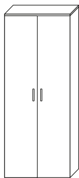
MPX-718 2 ante 2 ripiani 75x180x35/45cm
